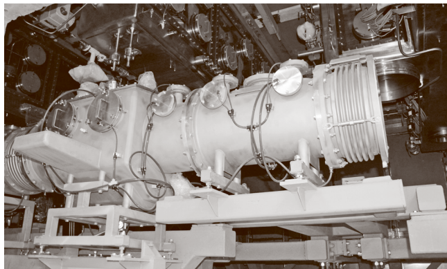
Участок карботермического синтеза: 110 тонн оборудования для получения нитридного топлива
