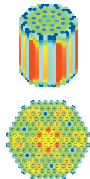
Активная зона реактора ВВЭР-1000
